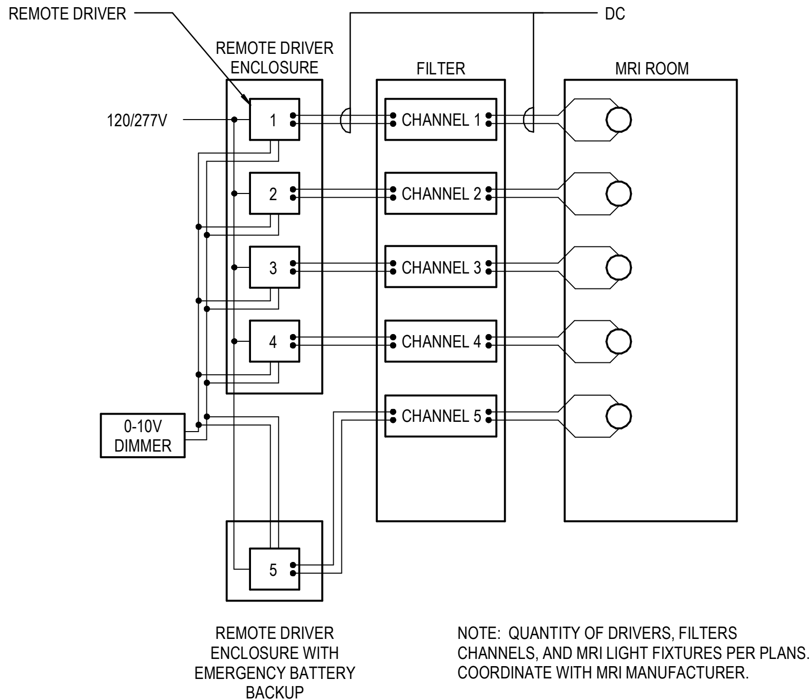
2 MRI LIGHTING SCHEMATIC N.T.S.
