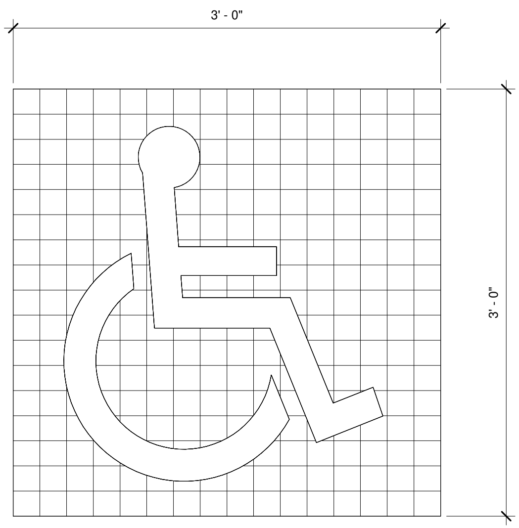
D1 ADA SYMBOL 1 1/2" = 1'-0"
