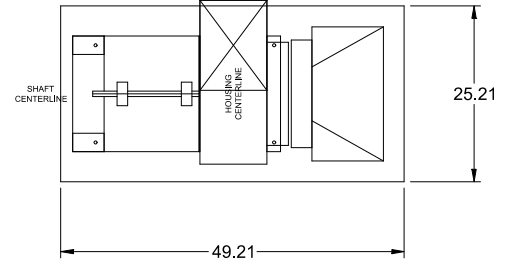
FAN FOOTPRINT
