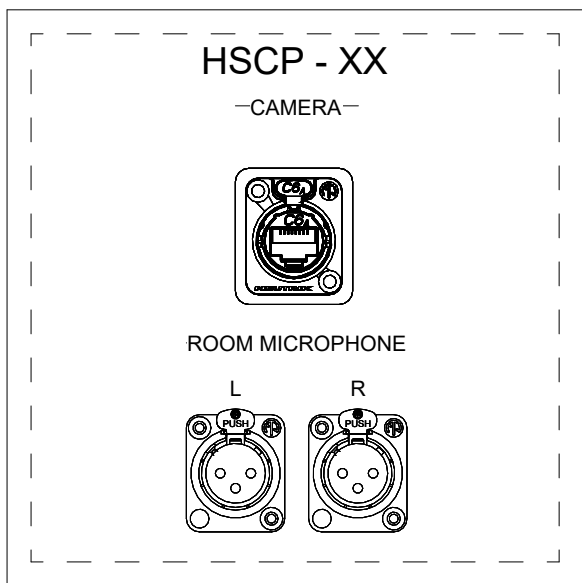
1 PANEL: HSCP - HOUSE PTZ CAMERA AV BOX TYPE: 6X6X6
