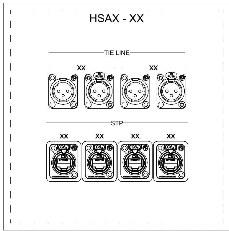
1 PANEL: HSAX - HOUSE AUX PANEL AV BOX TYPE: 8X8X6
