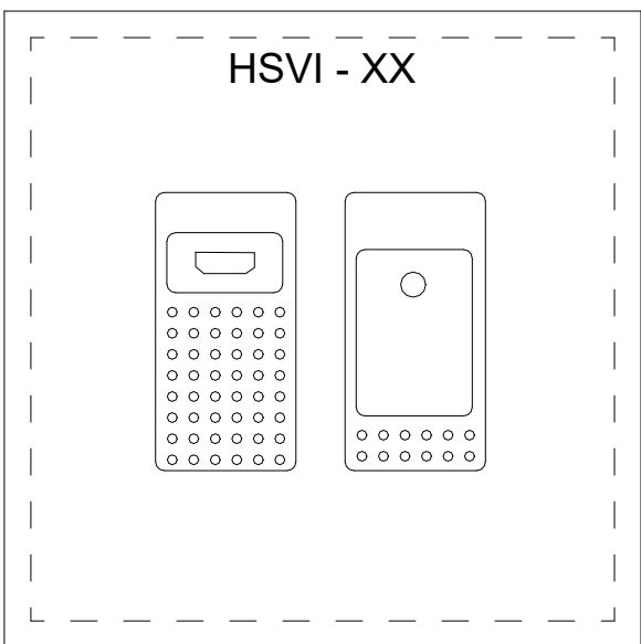
1 PANEL: HSVI - HOUSE VIDEO INPUT AV BOX TYPE: 6X6X6 WITH 2 GANG MUDRING
