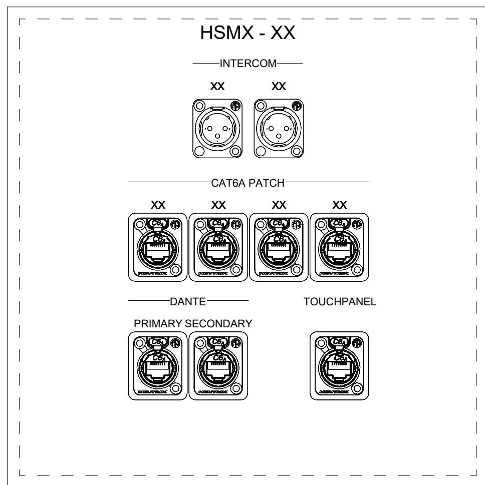
1 PANEL: HSMX - HOUSE MIX AV BOX TYPE: 10X10X6 AVIG , QUAD , CIRCUIT QTY: 2
