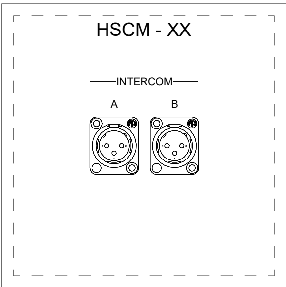
1 PANEL: HSCM - HOUSE INTERCOM AV BOX TYPE: 6X6X6
