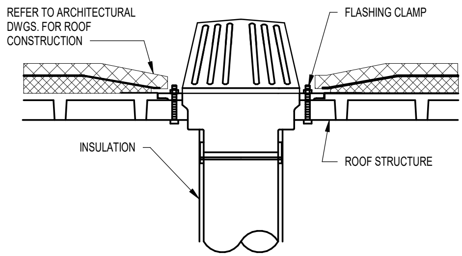
3 ROOF DRAIN SCALE: N.T.S.
