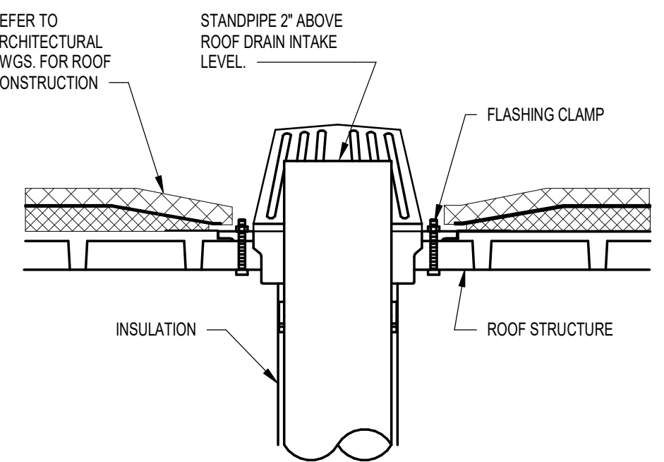
2 OVERFLOW DRAIN SCALE: N.T.S.
