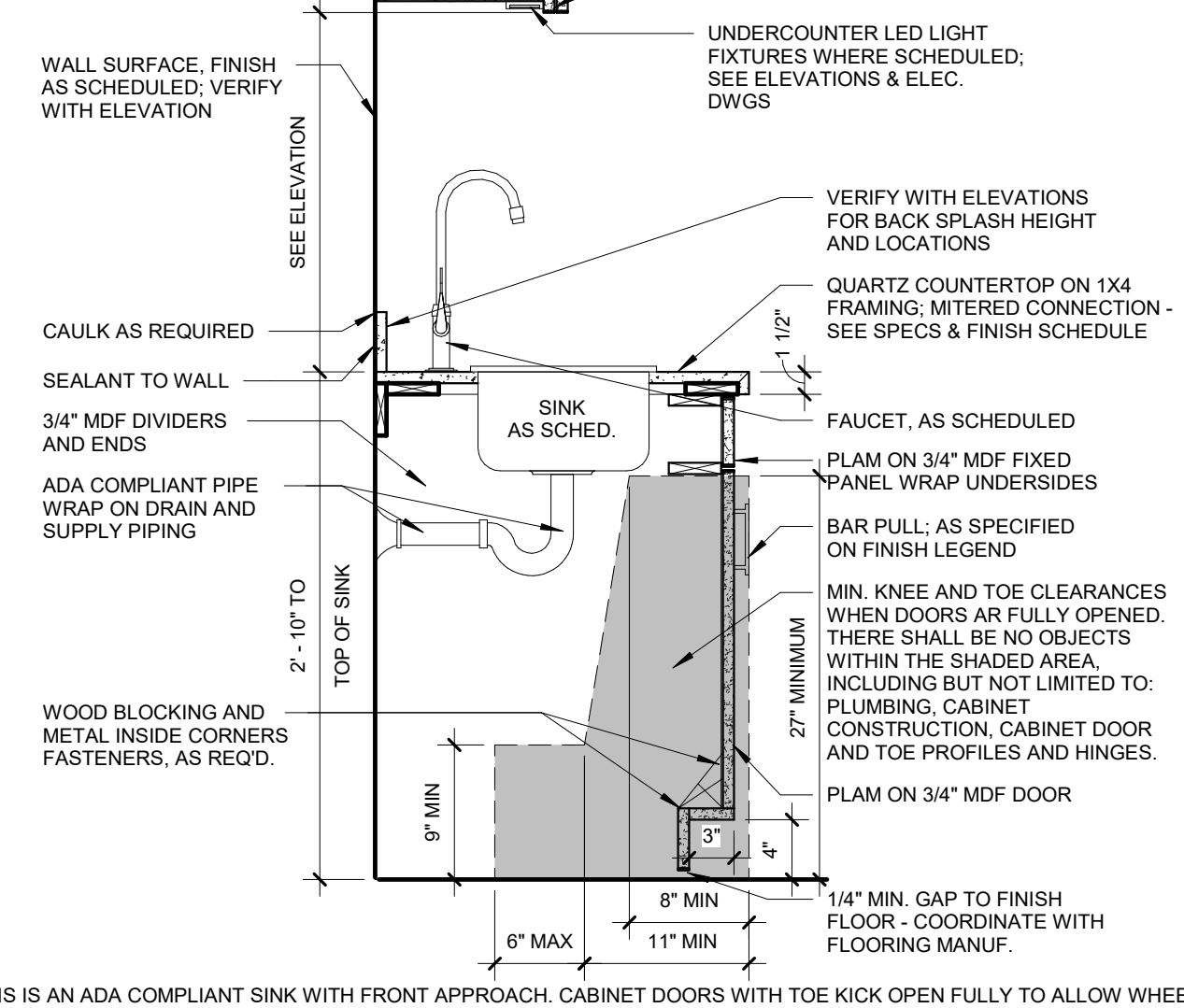
12 WALL & BASE CABS - ADA DOOR & SINK - QZ CTR 1" = 1'-0"
