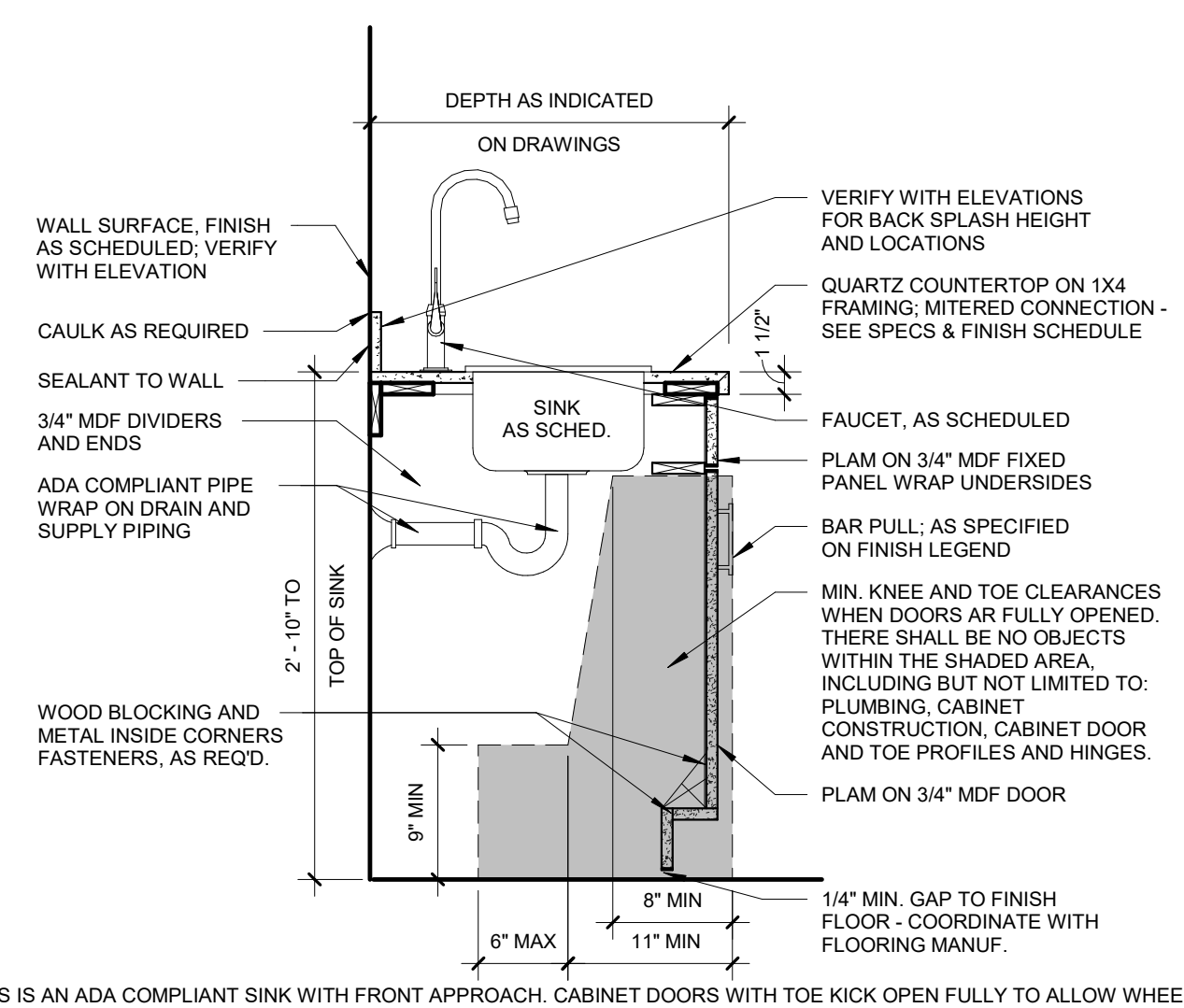
11 BASE CABS - ADA DOOR & SINK - QZ CTR 1" = 1'-0"
