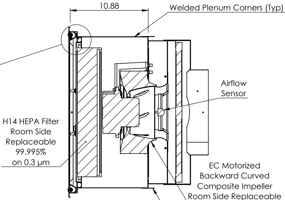
SECTION A-A SCALE 1 : 8
