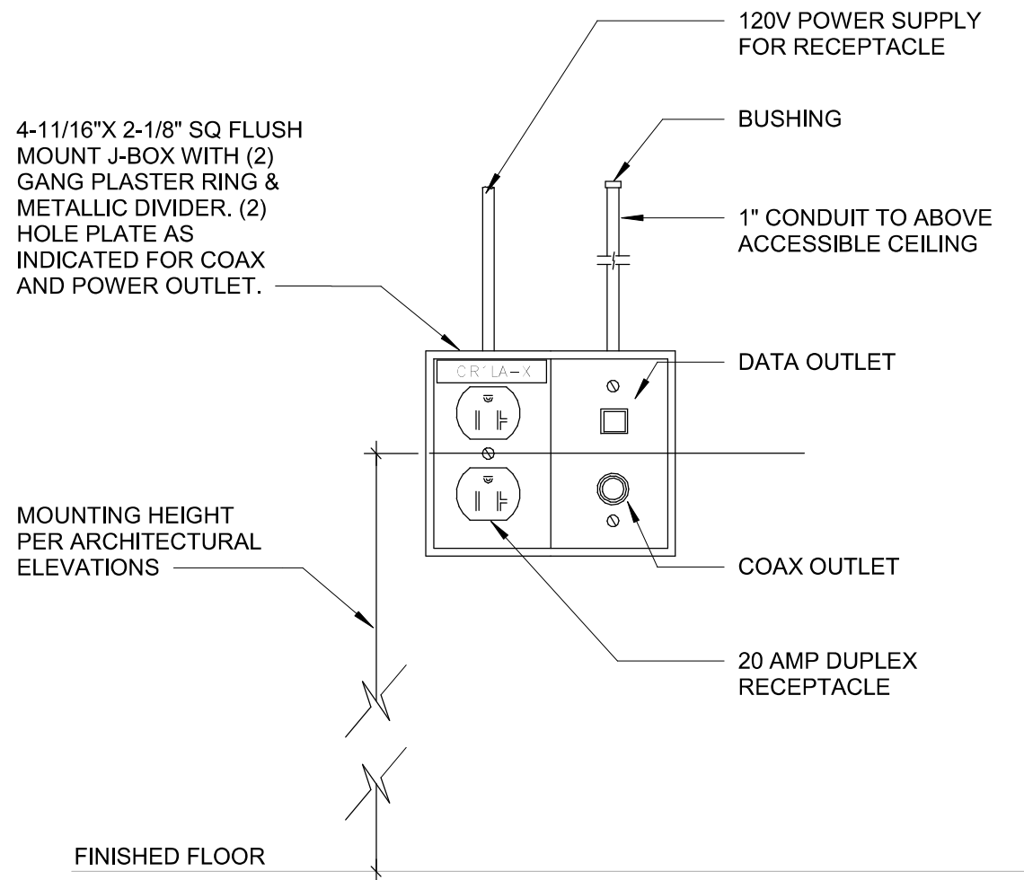
A5 POWER/TV OUTLET NO SCALE
