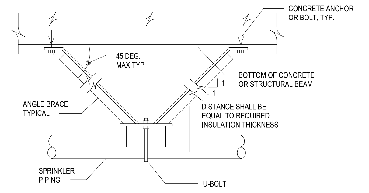
LONGITUDINAL BRACE DETAIL
