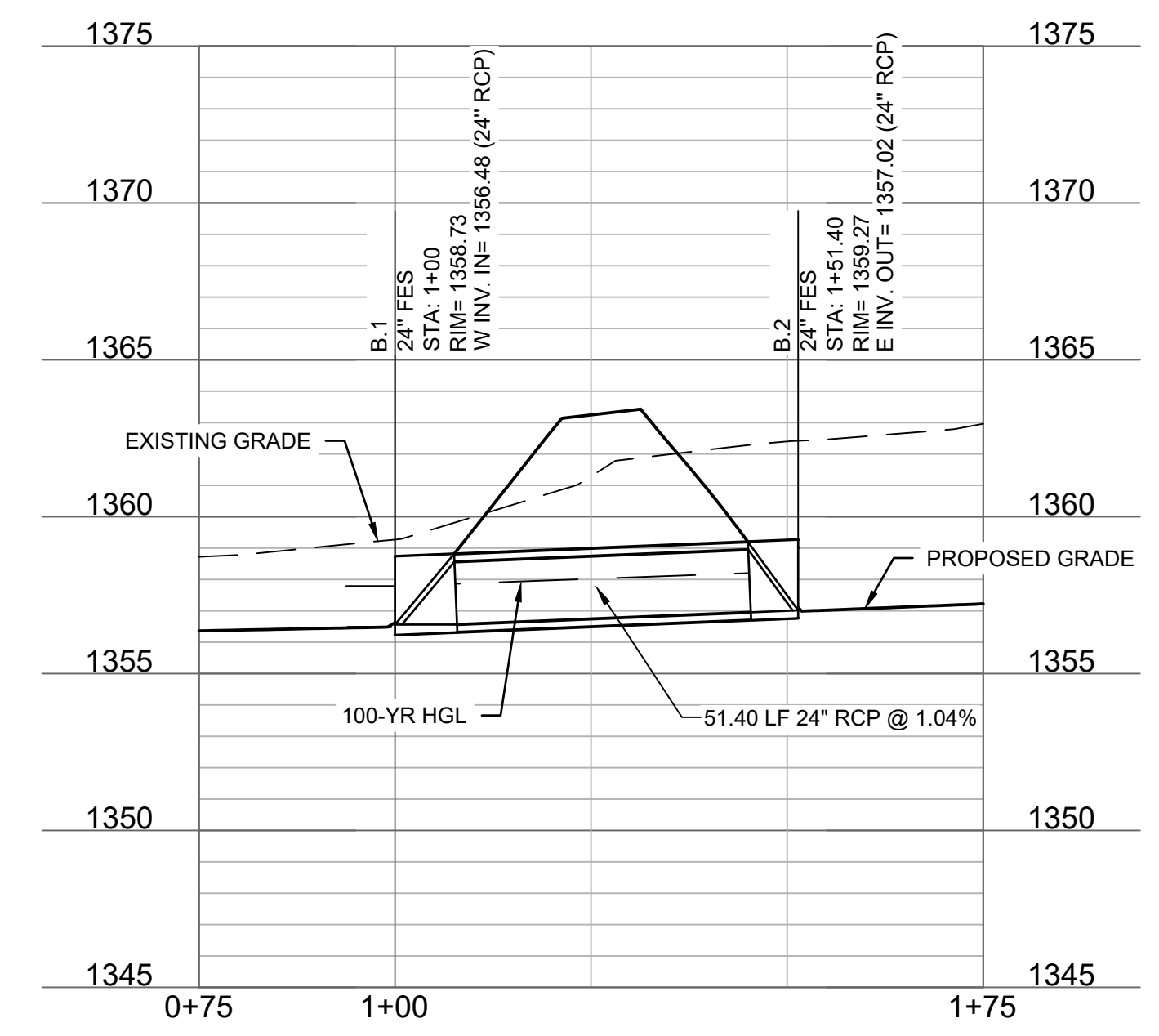
STORM LINE B (0+75 - 1+75)
