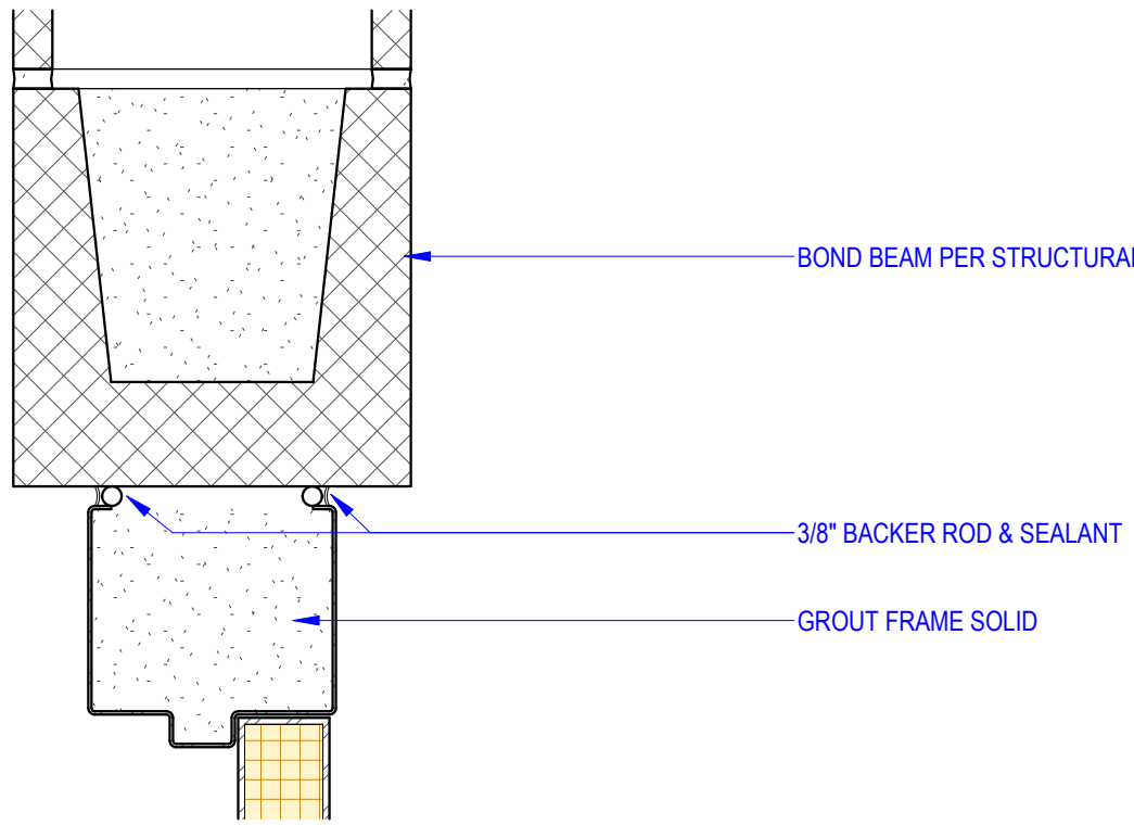
D3 DOOR HEADER 3" = 1'-0"
