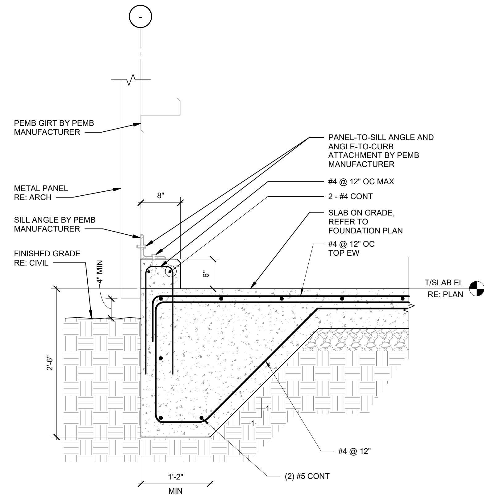
A3 THICKENED SLAB EDGE SCALE 1" = 1'-0"
