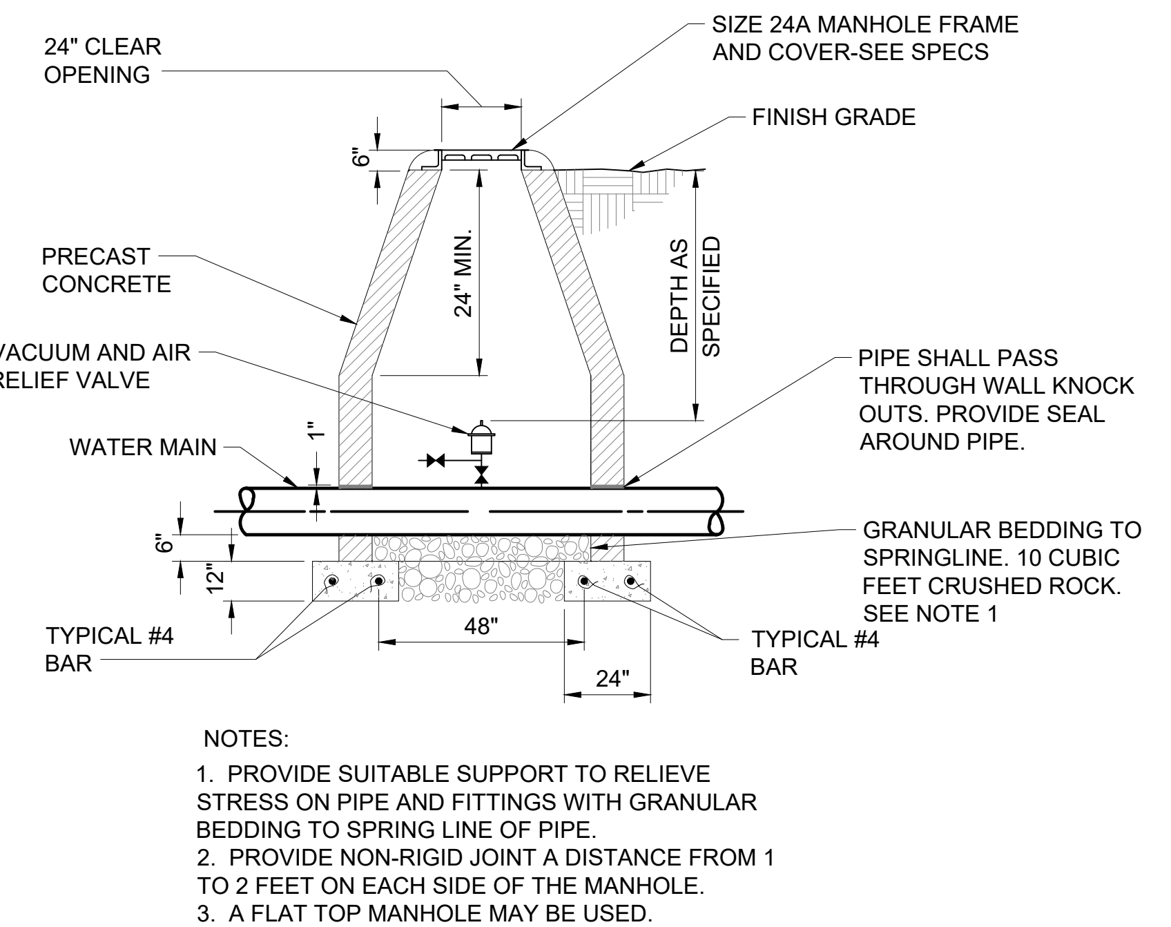
B5 AIR VACUUM SCALE N.T.S.
