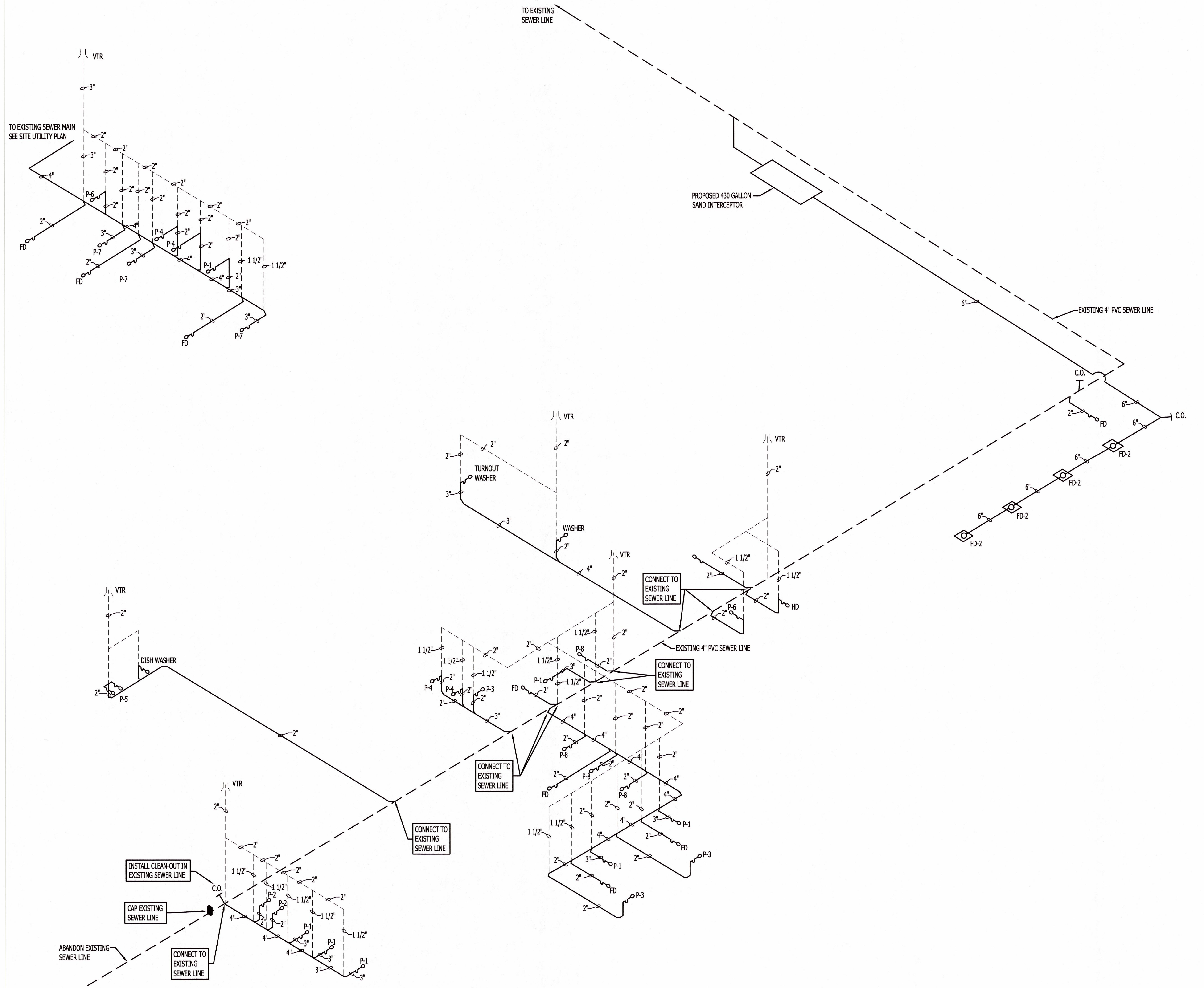
SANITARY SEWER RISER N.T.S.
