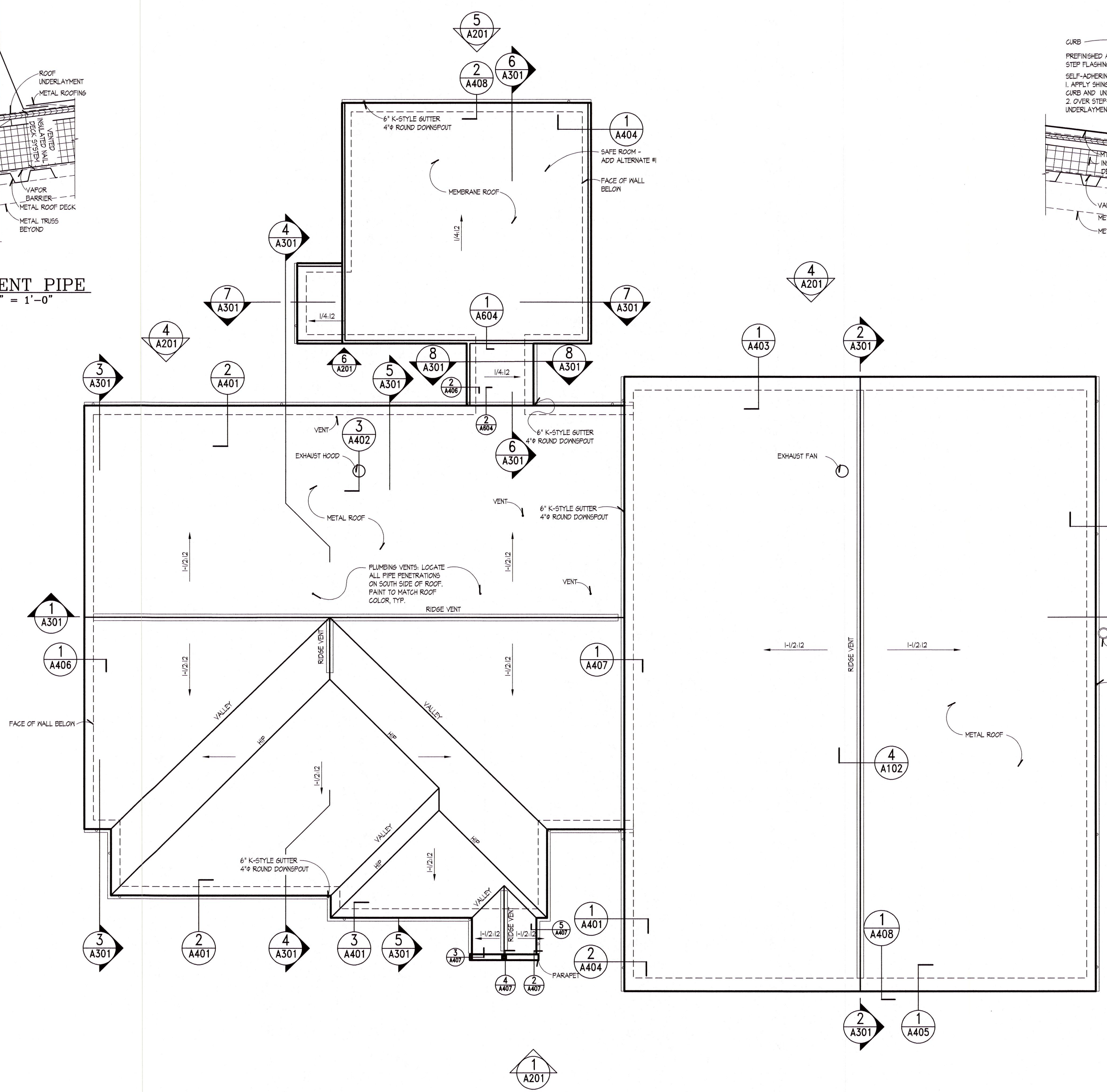
1 ROOF PLAN A102 SCALE: 1/8" = 1'-0"
