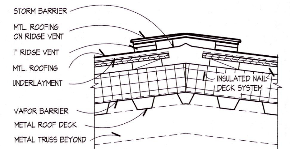
4 METAL ROOF CAP A102 SCALE: 1 1/2" = 1'-0"
